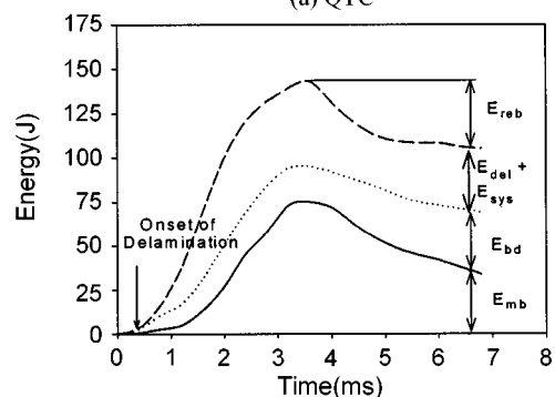
(b) UD
